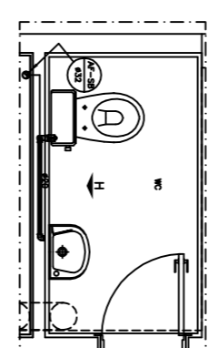
DETALHE-6 - SOBRE LOJA
