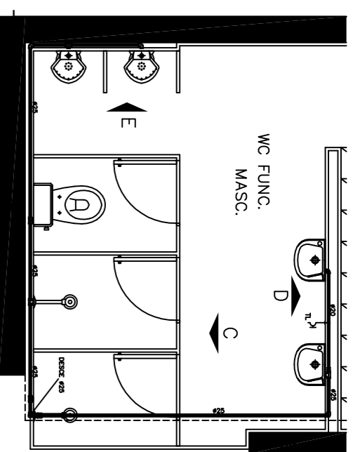
DETALHE-2 1º SUBSOLO
